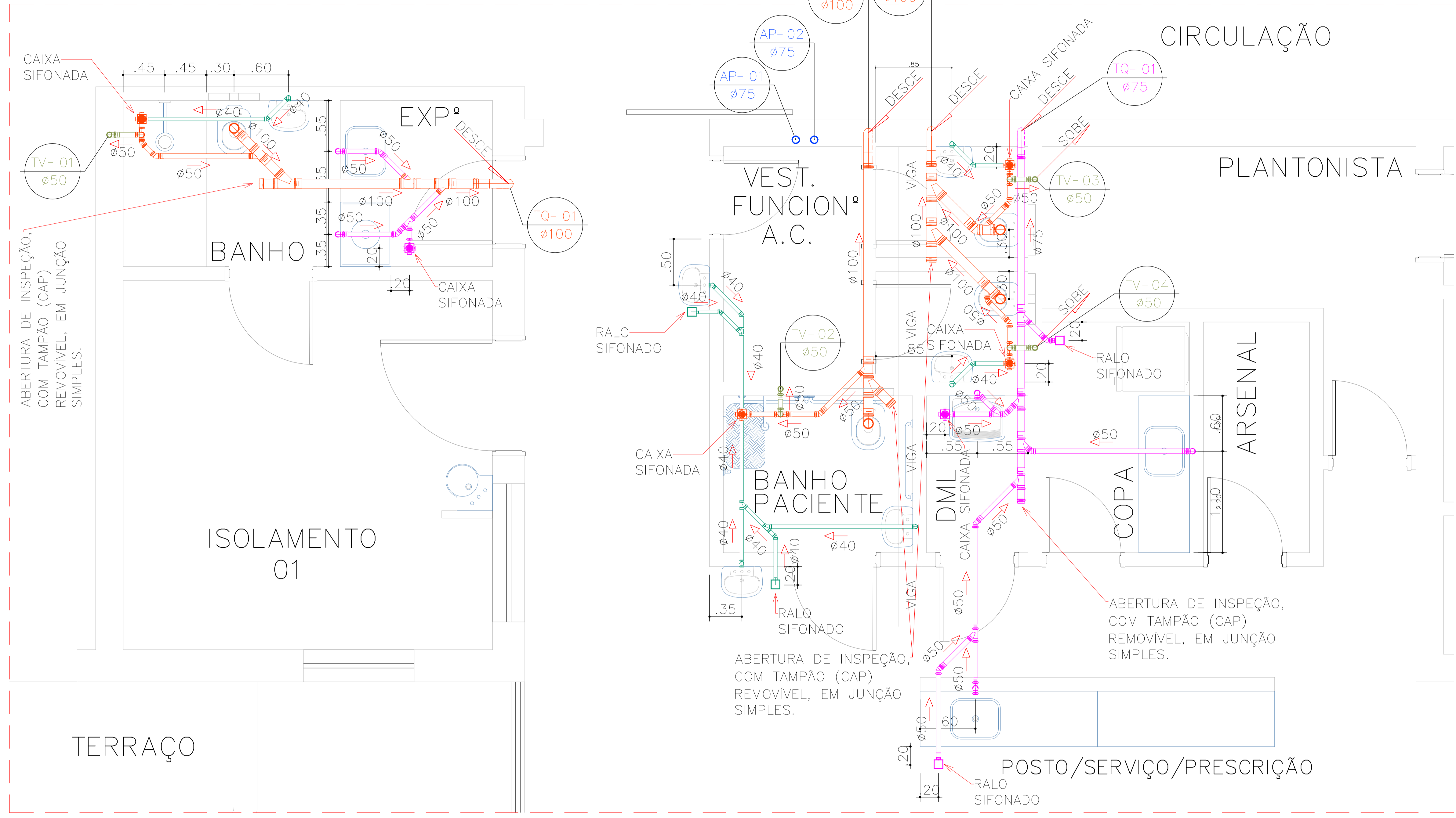
PLANTA PAVIMENTO SUPERIOR ESCALA 1:25
